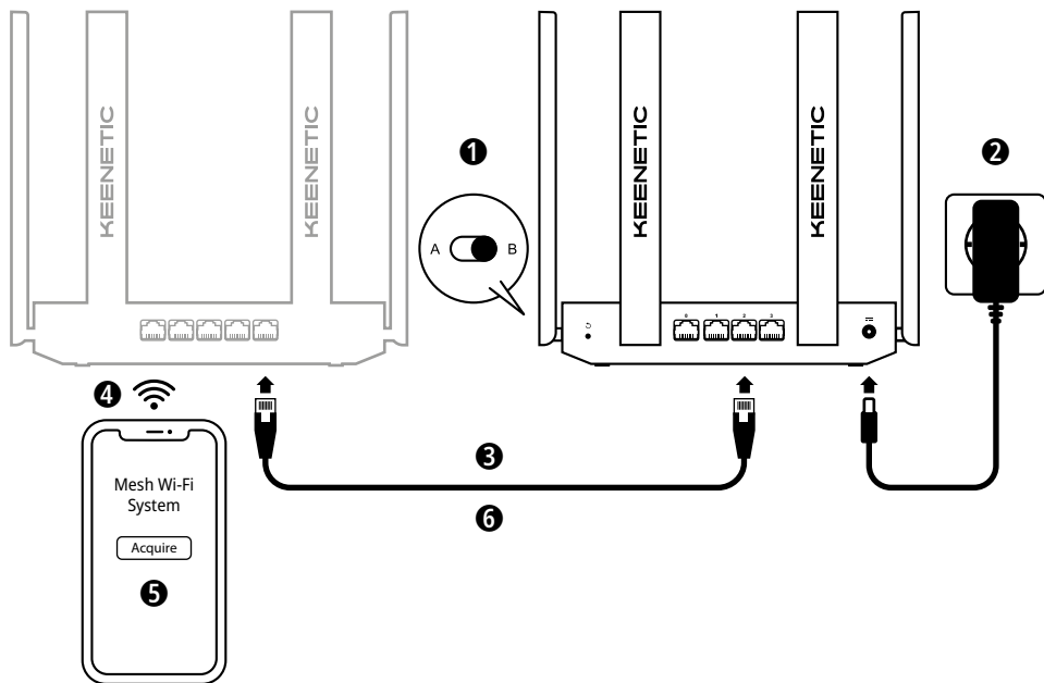
B. Rozšíření pokrytí stávající sítě Podrobnosti na obrázku se mohou lišit od vašeho konkrétního zařízení.
