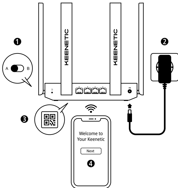
A. Свързване на основния Ви рутер към интернет Изображението може да се различава от вашето конкретно устройство.
