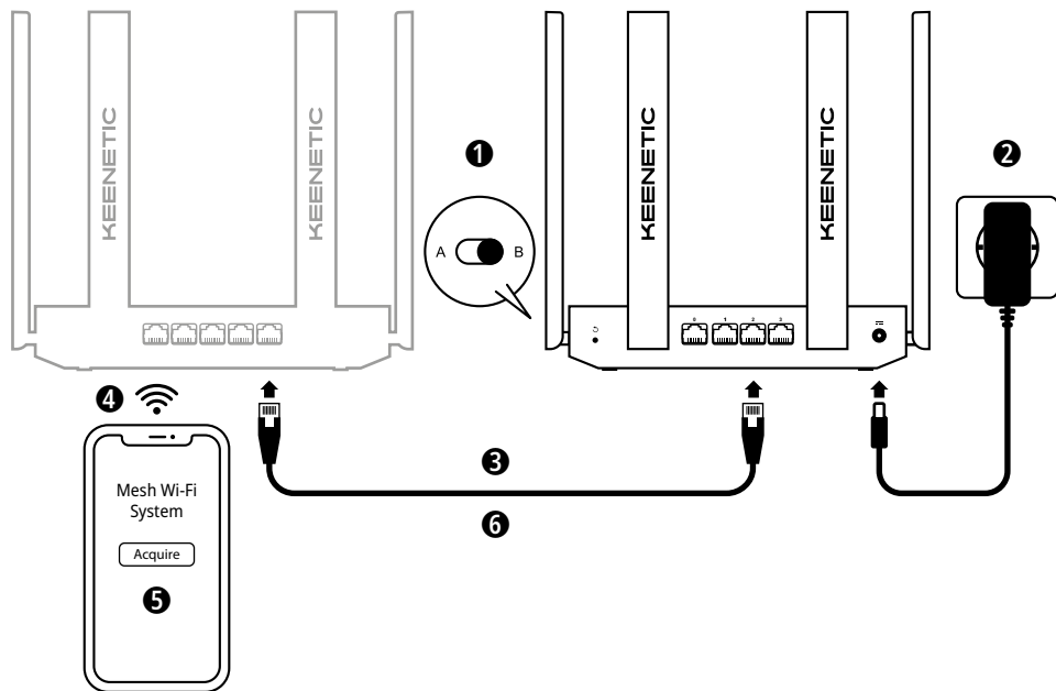
B. Proširivanje doseg postojće mreže Slika se može razlikovati od vašeg konkretnog uređaja.
