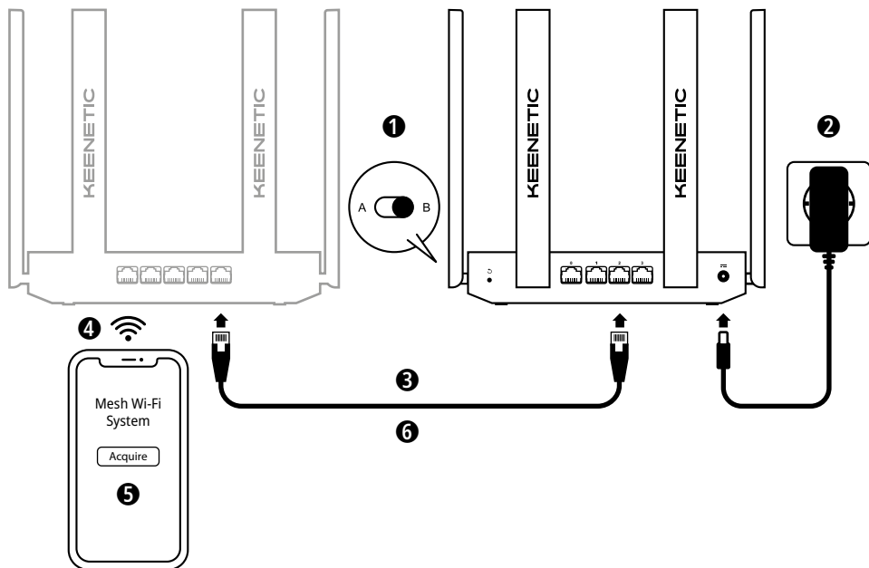
B. Proširenje dometa postojeće mreže Slika može da se razlikuje od vašeg uređaja.
