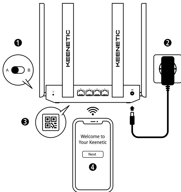
A. Conexión del router principal a Internet Los datos de la imagen pueden ser distintos a los de su dispositivo.
